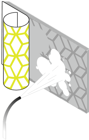
5 Kalvo poistetaan helposti betoniosasta ja betoni puhdistetaan painepesurilla.
